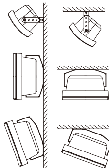
2. 通过支架挂壁或天花板安装
