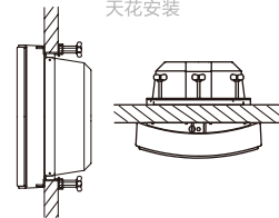
4. 组合吊装方式
