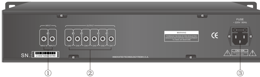
① A、B通道信号源输入 ②通道1至通道6信号输出 ③电源插座
